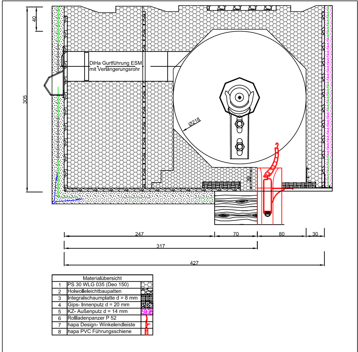
Bild 2 Schnittzeichnung
